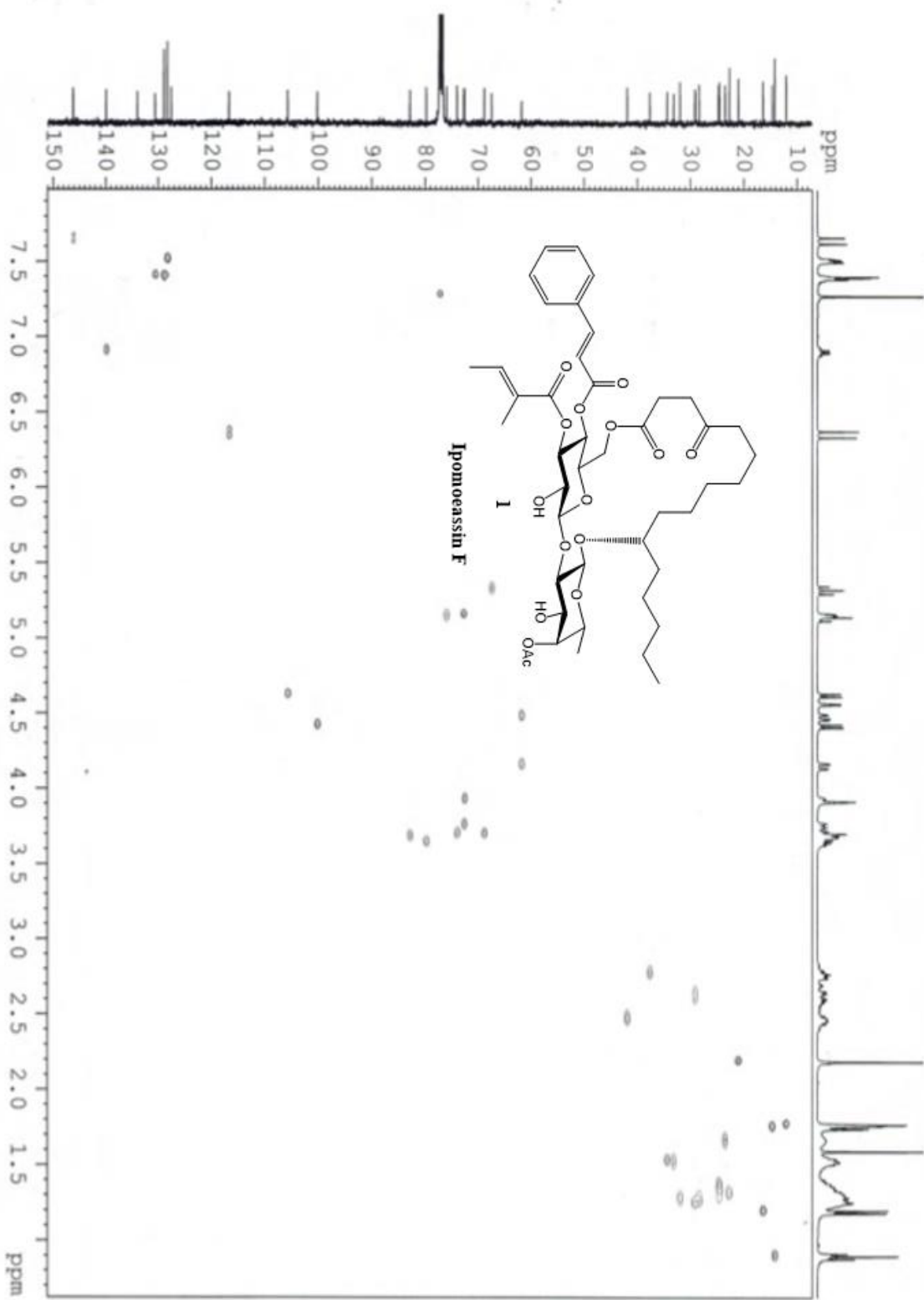
LW-|pomo-F-2-1-1704_|Ipomoassin F HSQC 400 LW
