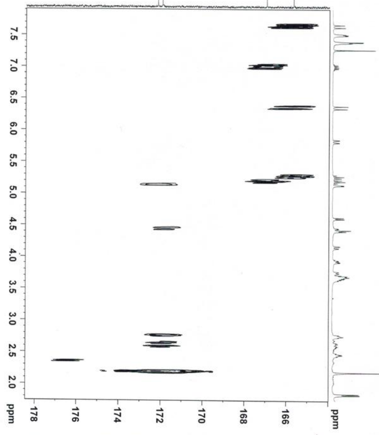
LW-IPom-F-2-20-170426 HMBC in CDCl3 400 NMR
